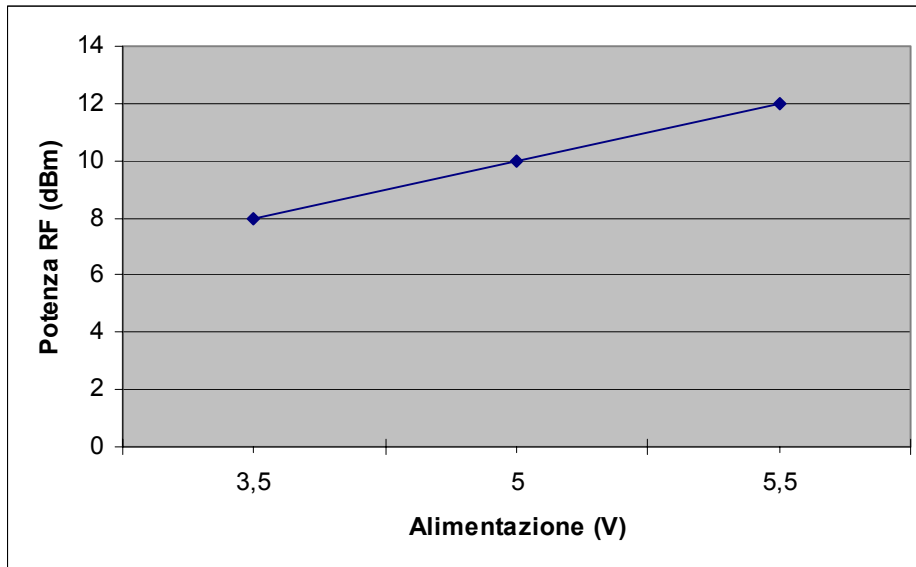
Fig. 3 Andamento della potenza RF in funzione della tensione di alimentazione
